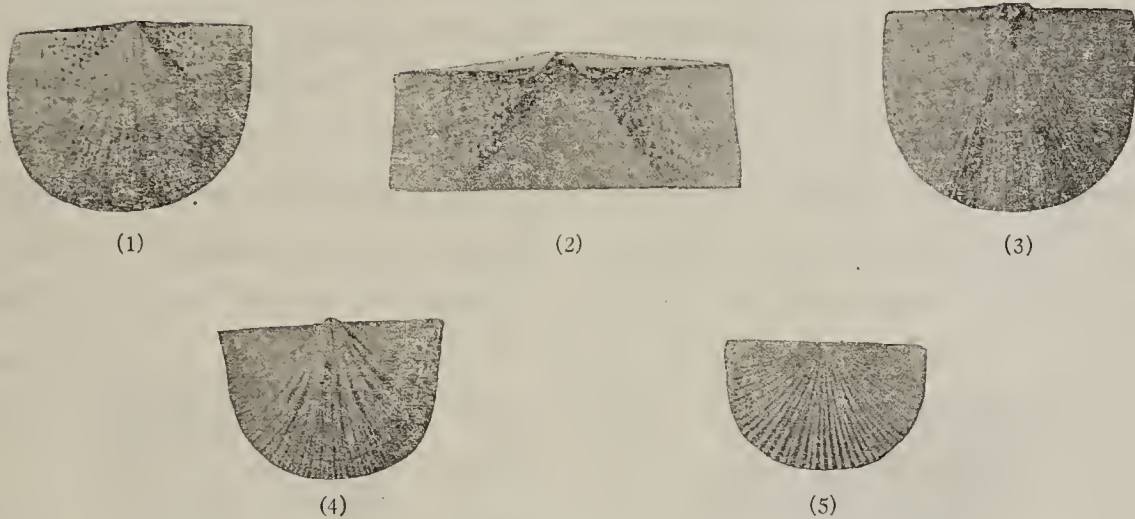
Fig. 1 — Molde internal da valva ventral ; Fig. 2 — Area cardinal ventral augmentada ; Fig. 3 — Interior da valva dorsal ; Fig. 4 — Molde da esculptura da valva ventral. Fig. 5 — Exterior da valva dorsal.
